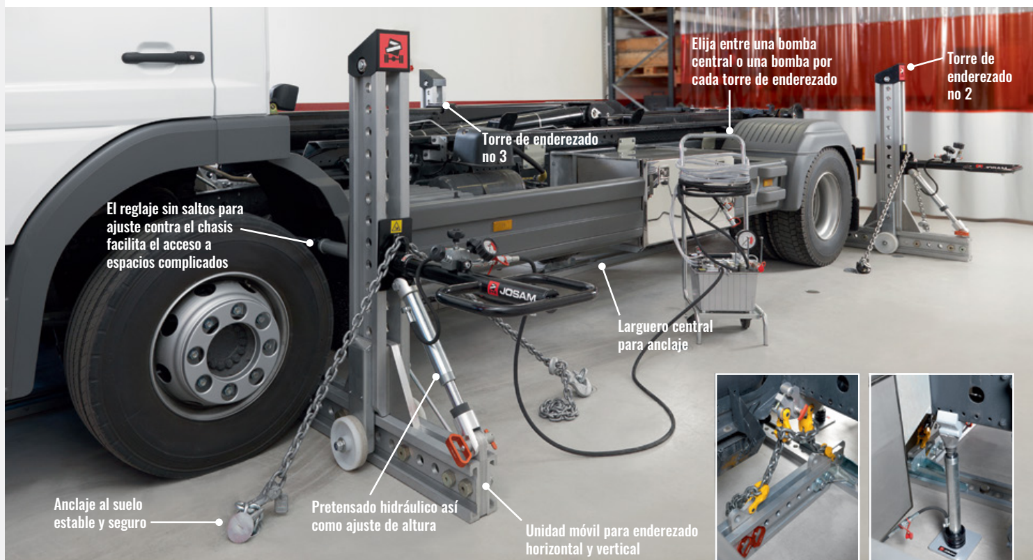
Torre de enderezado instalada como apoyo vertical
