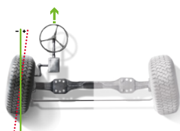
Centrage du boîtier de direction
